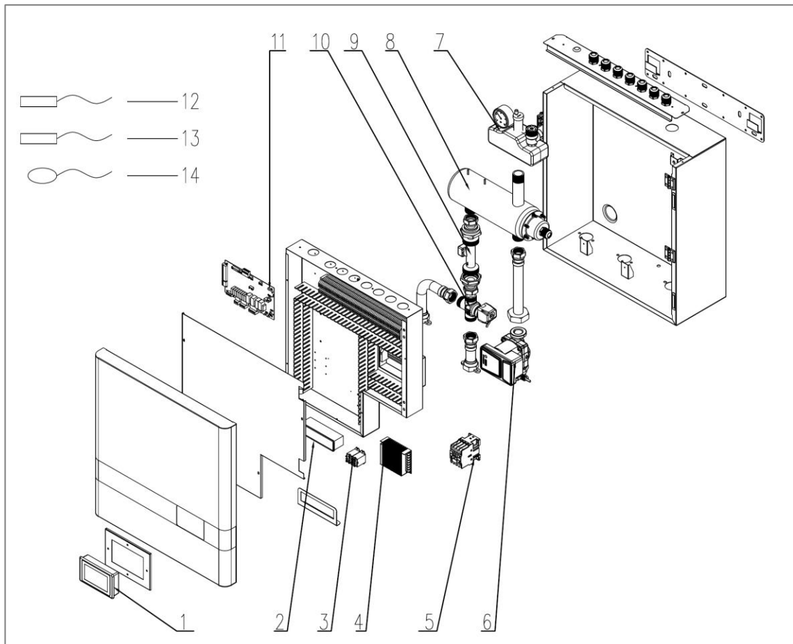
Abbildung 9: Einzelkomponenten des Innengeräts (MB700008 und MB700015)
