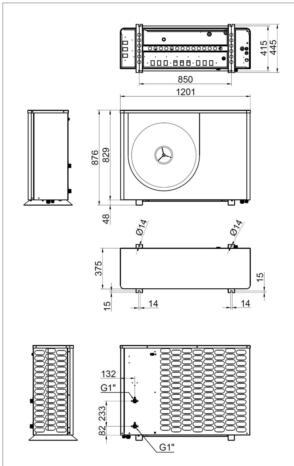
Abbildung 17: Abmessung Außengerät MB70008A – Maße in mm
