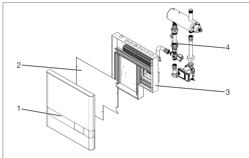
Abbildung 24: Die Elektronik befindet sich unter der Abdeckung
