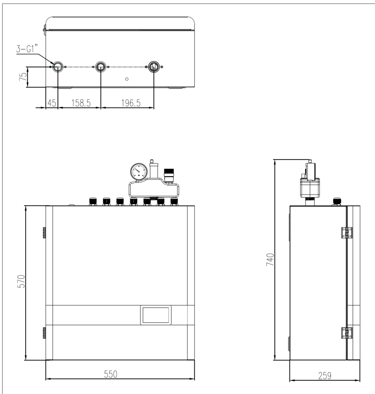
Abbildung 16: Abmessung Innengerät – Maße in mm
