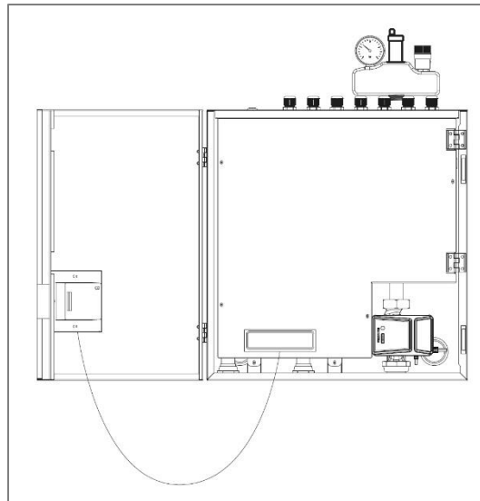
Abbildung 26: Die Elektronik befindet sich unter der Abdeckung
