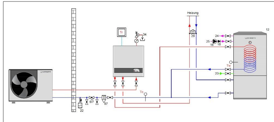
Abbildung 12: Wärmepumpe mit Trinkwasserspeicher und Heizungsanschluss
