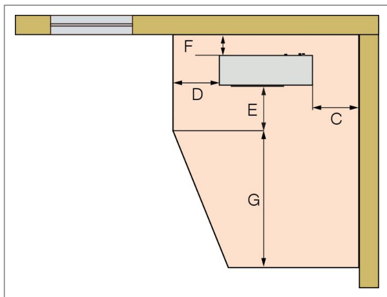
Abbildung 5: Aufstellung an einer Gebäudeecke rechts, auch Spiegelverkehrt gültig mit Gebäudeecke links.
