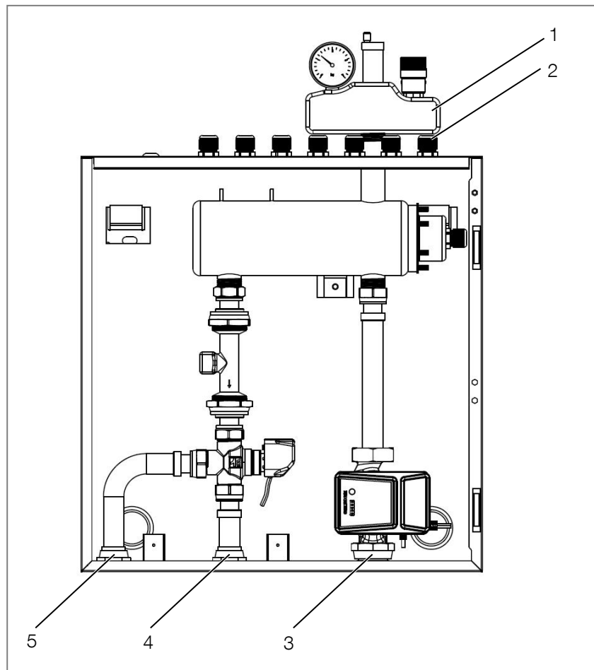
Abbildung 19: Anschlüsse Innengerät (MB700008 und MB700015)
