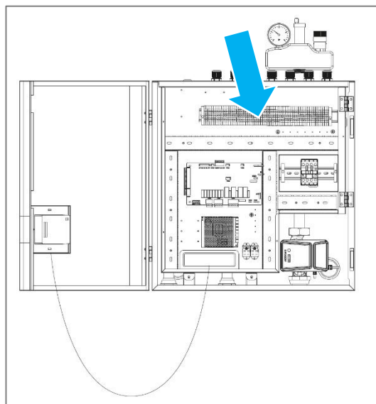
Abbildung 25: Position der Klemmleiste auf der Ebene 3
