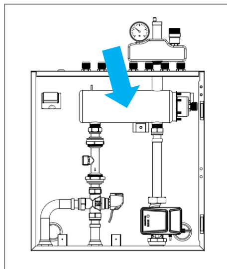
Abbildung 27: Elektrische Heizung
