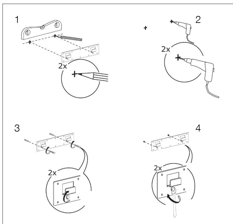
Abbildung 14: Montageplatte befestigen
