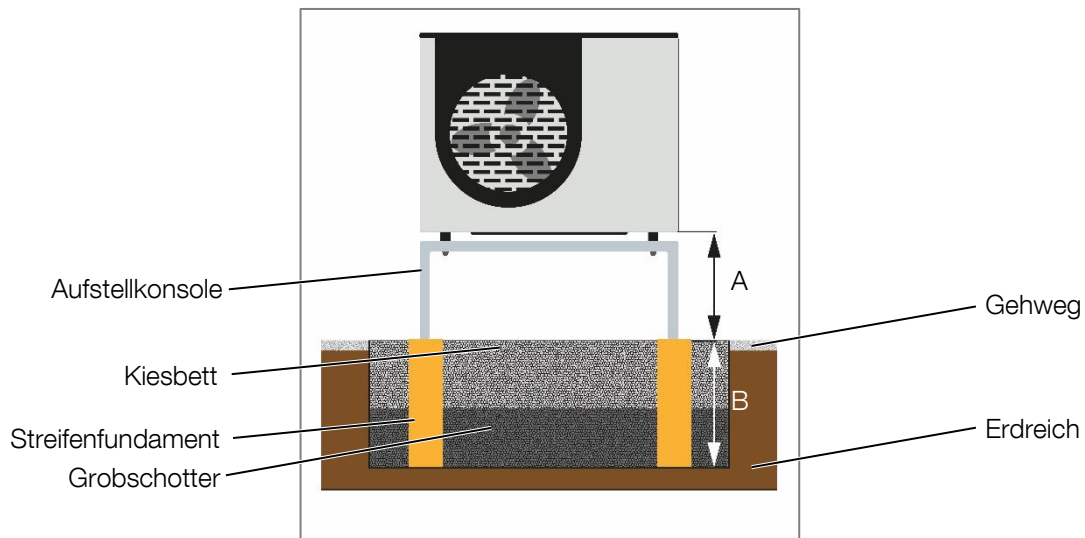
Abbildung 6: Fundament mit Grobkies
