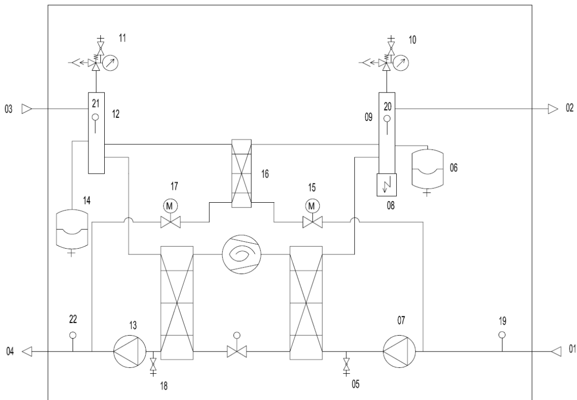
Wärmepumpe EcoTouch 5029Ai NC
