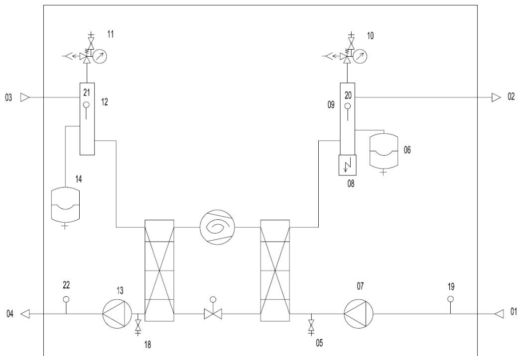
Wärmepumpe EcoTouch 5029Ai NC
