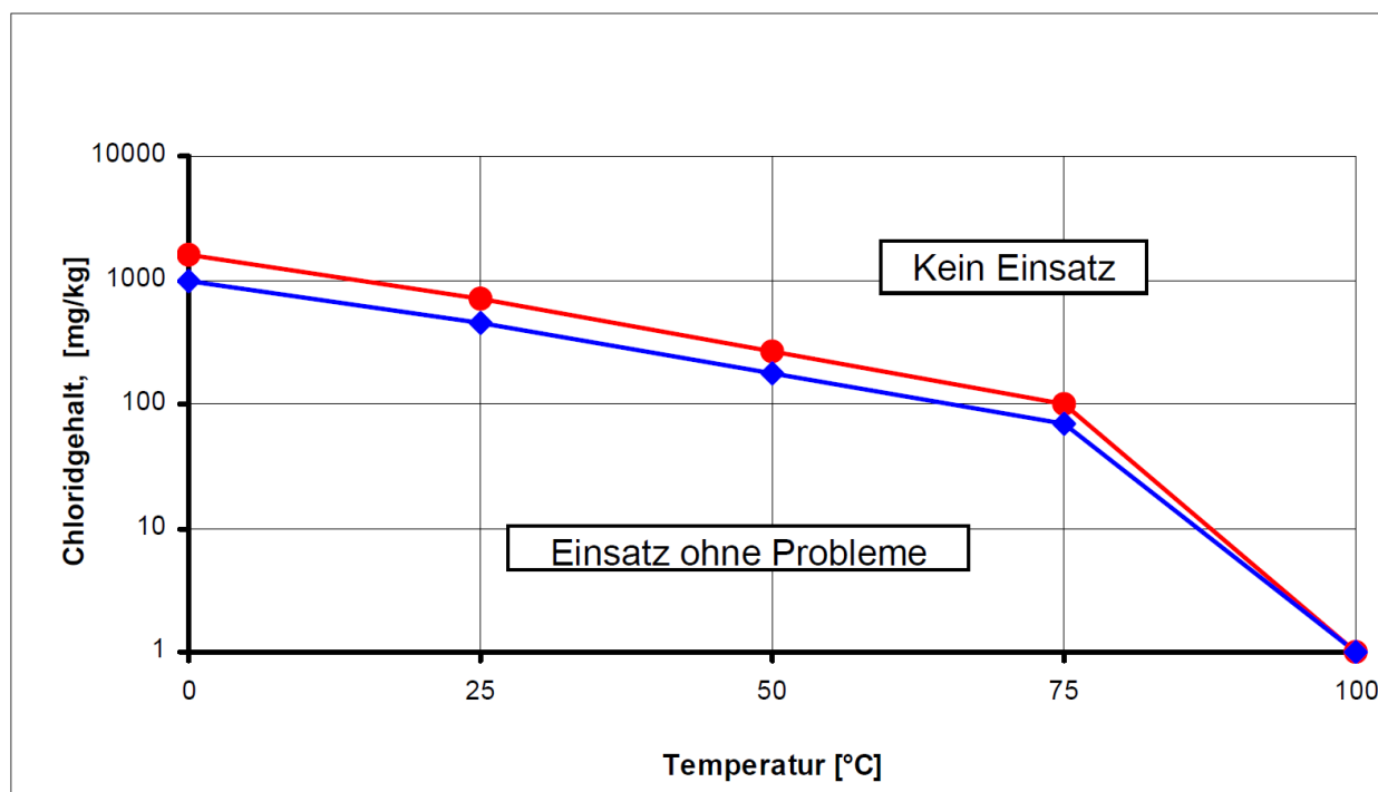
Abbildung 5: Zulässiger Chloridgehalt in Abhängigkeit der Temperatur
