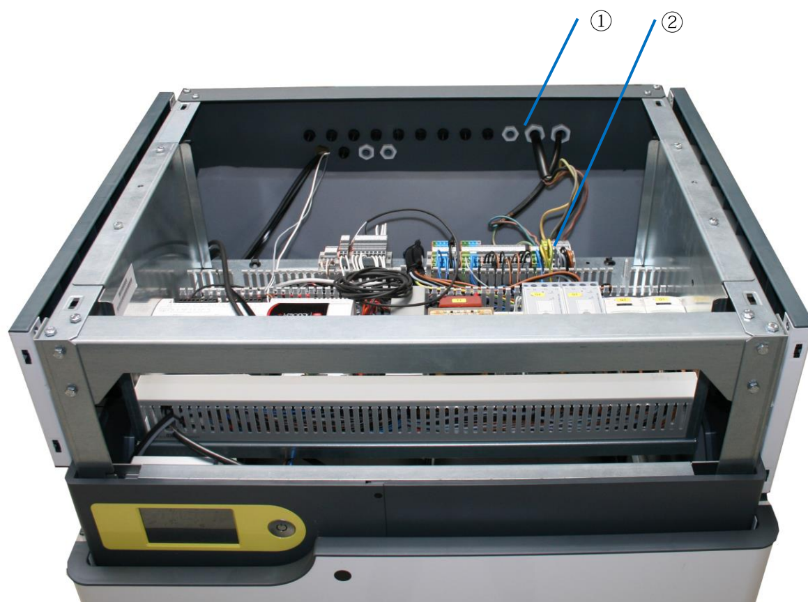
Abbildung 3: EcoTouch DS 5050T(Draufsicht, geöffnet)
