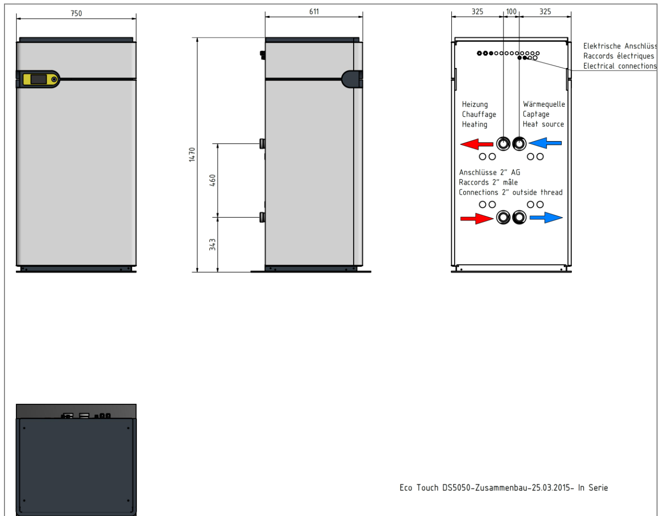
Abbildung 4: Anschlüsse EcoTouch DS 5050T(Rückseite)
